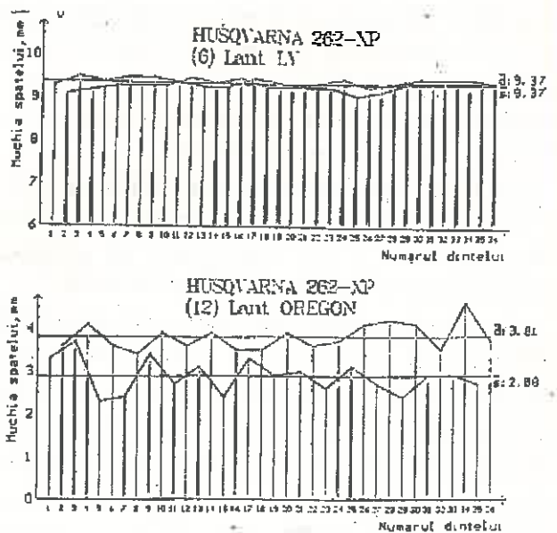
Fig. 2. Variația lungimii muchiei spatelui la un lanț nou (6) și un lanț uzat (12). (Length variation of the back margin by a new chain (6) and a worn-out one (12)).
