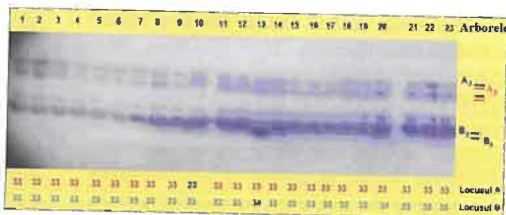
Fig. 1. Zimograma locilor genici Idh-A și Idh-B pentru arbori analizați în Munții Poiana Ruscă
